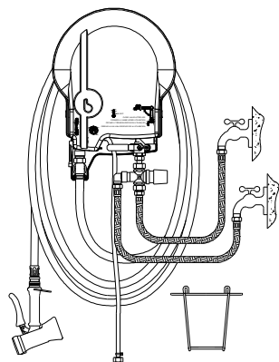
MITIGEUR THERMOSTATIQUE PMITI00002
