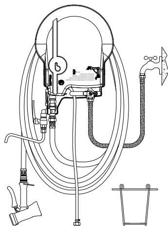
KIT DILUTION AVEC BEC VERSEUR INOX PKITA00011
